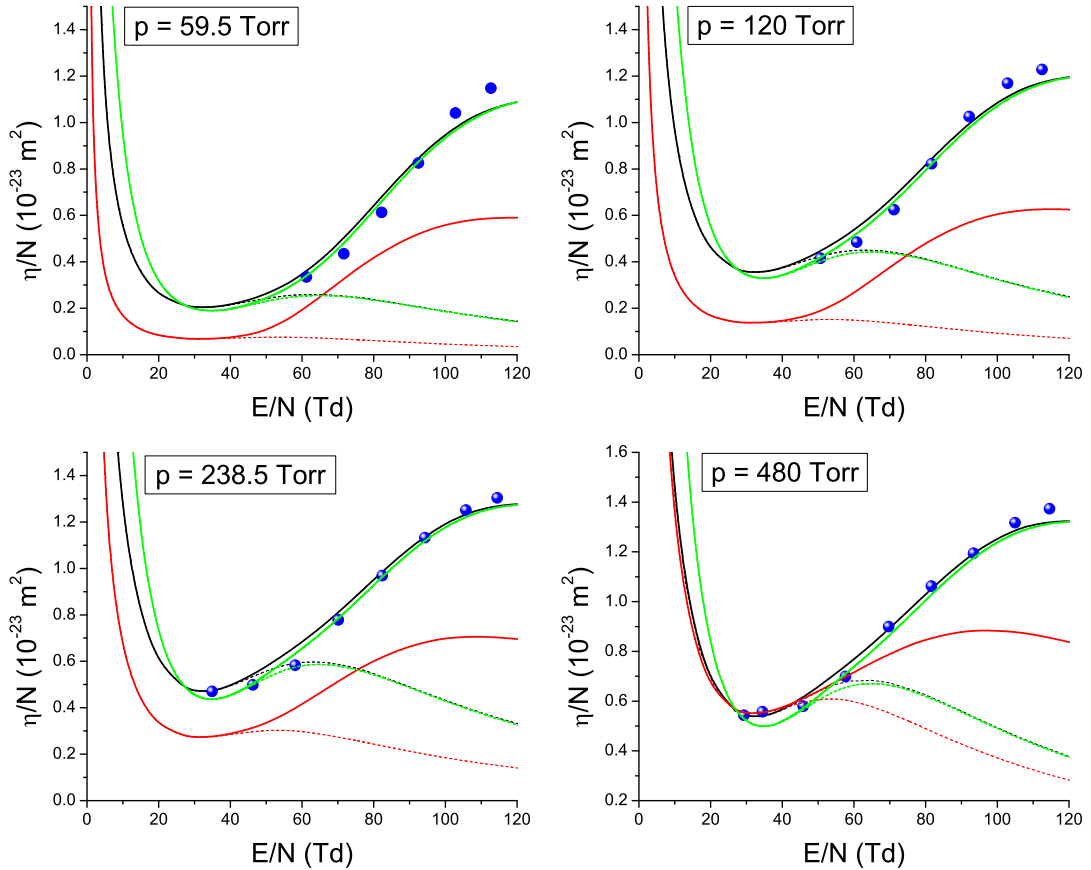
Slika 5.27: Totalni i trojni koeficijenti zahvata u funkciji E/N na različitim pritiscima za elektrone u C_2H_2F_4 . Crne linije: Monte Karlo rezultati, Crvene linije: MAGBOLTZ rezultati, Zelene linije: BOLSIG+ rezultati, Pune linije: Koeficijent za ukupni zahvat, Isprekidane linije: Koeficijent za trojni zahvat, Plavi okrugli simboli: Eksperimentalni podaci Basile i saradnika.
