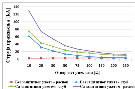
Слика 5.9 – Утицај заштитног ужета и мјеста пражњења на минималну амплитуду струје која узрокује испад 110 kV вода из погона
