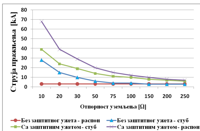
Слика 5.6 – Утицај заштитног ужета и мјеста пражњења на минималну амплитуду струје која узрокује испад 35 kV вода из погона
