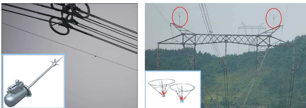
Слика 3.23 – а) Иглица за заштитно уже и б) громобранске хватаљке са контролисаним празњење постављене на врху стуба 500 kV вода [131]
