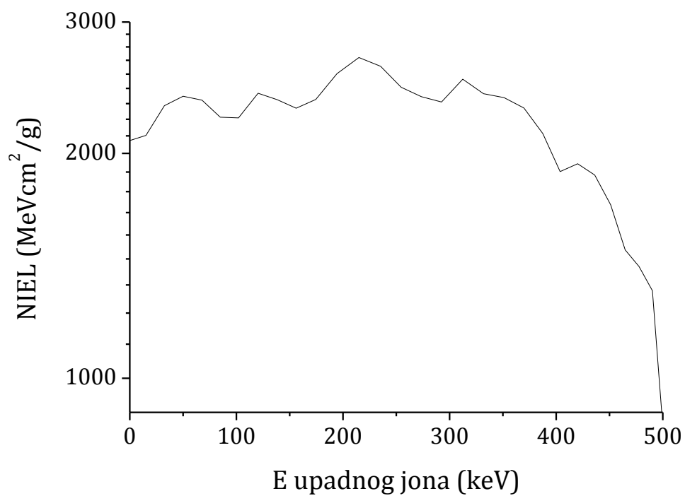
Slika 6.28d. Nejonizujući energetske gubici za Fe jone u ASS materijalu u zavisnosti od energije.
