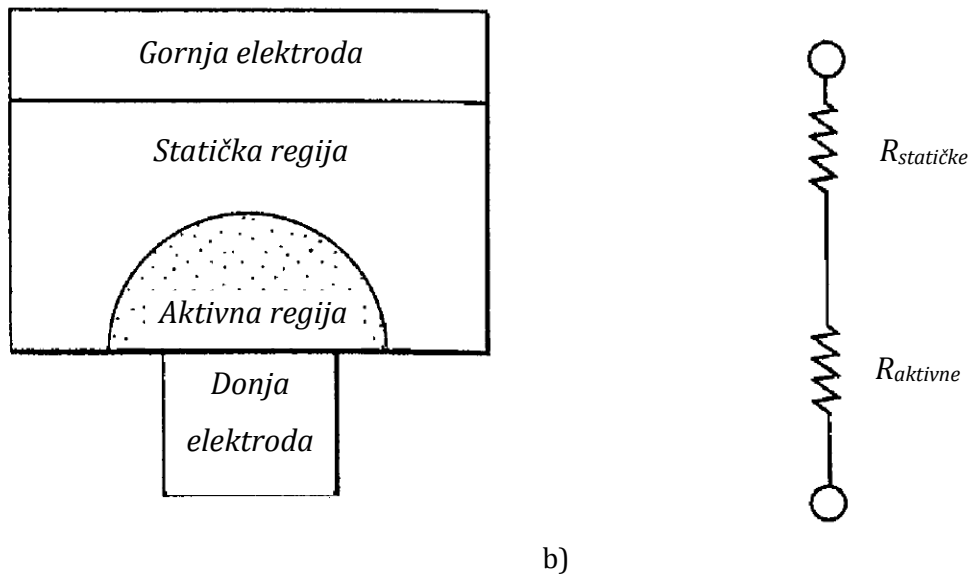
Slika 3.9. a) Tipična fazno promenljiva ćelija u RESET stanju, b) serijski vezane otpornosti aktivne i statičke regije
