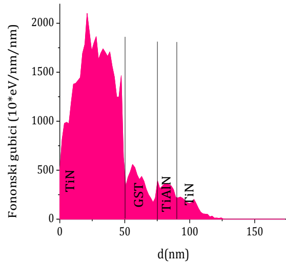
Slika 6.13e. Fononski energetska gubici nastali od upadnih Ar jona i izmeštenih atoma čelije FPM-a.
