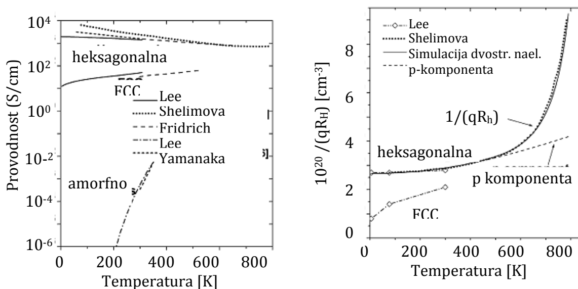
Slika 3.25. Temperaturska zavisnost a) prvodnosti i b) 1/(qR_H) u GST materijalu [44]
