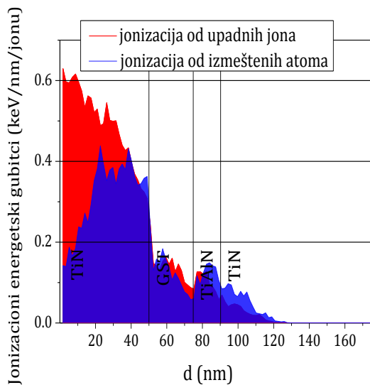
Slika 6.13a. Transport Ar jona kroz fazno promenljivu ćeliju sa GST slojem.
