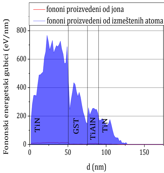
Slika 6.13d. Fononski energetska gubici nastali od upadnih Ar jona i izmeštenih atoma čelije FPM-a.
