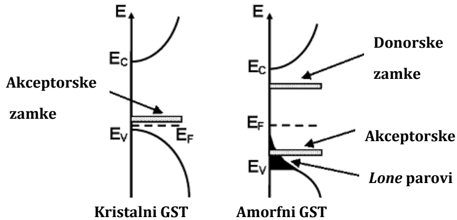
Slika 4.8 Energeski dijagram kristalnog i amornog GST materijala [18]
