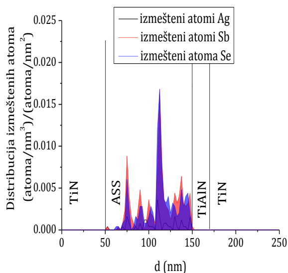
Slika 6.18c. Distribucija izmeštenih atoma Ag, Sb i Se.
