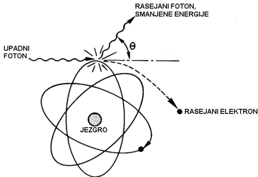
Slika 2.4. Komptonovo rasejanje
