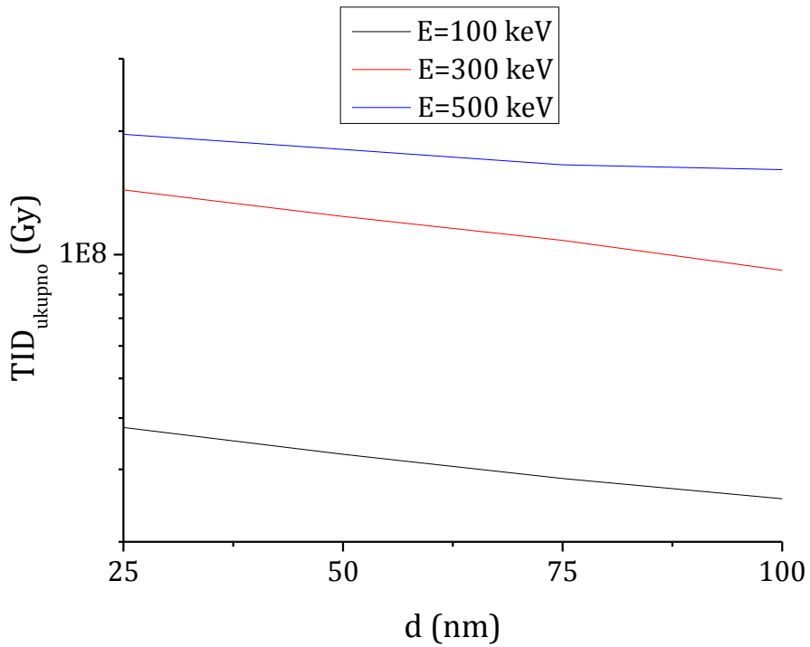
6.31a. Ukupna jonizacijska doza u celoj ćeliji FPM-a u zavisnosti od debljine ASS sloja za različite energije upadnih Ar jona.
