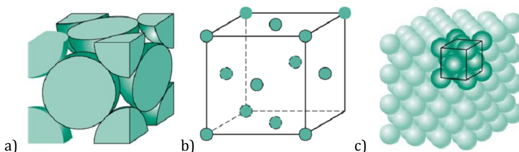
Slika 3.19. Šematski prikaz površinski centrirane kristalne rešetke a) prikaz atomski čvrstih sfera, b) redukovani prikaz rešetke, c) prikaz u celini
