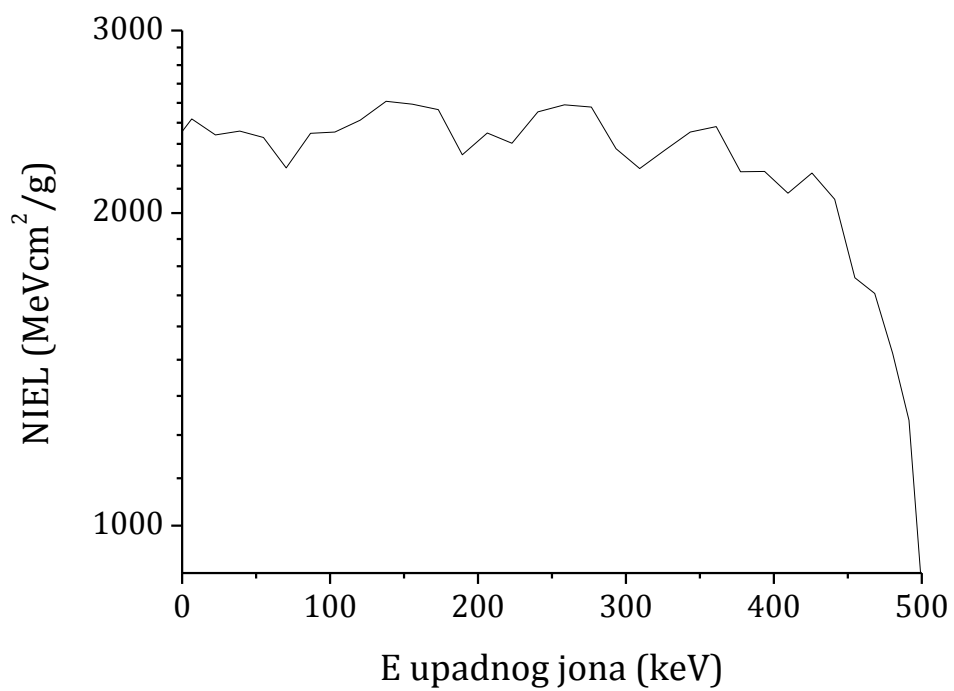
Slika 6.12d. Nejonizujući energetske gubici za Fe jone u GST materijalu u zavisnosti od energije jona.
