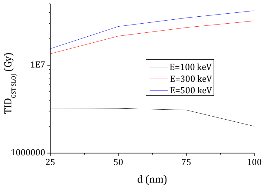
Slika 6.31b. Ukupna jonizacijska doza u ASS sloju u zavisnosti od debljine ASS sloja za različite energije upadnih Ar jona.
