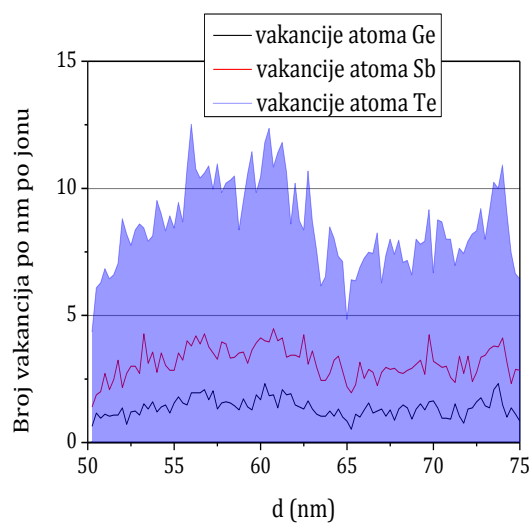
Slika 6.9g. Distribucija nastalih vakancija atoma Ge, Sb i Te u GST sloju.
