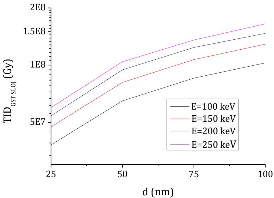
Slika 6.23b. Ukupna jonizacijska doza u ASS sloju u zavisnosti od debljine ASS sloja za različite energije upadnih alfa čestica.
