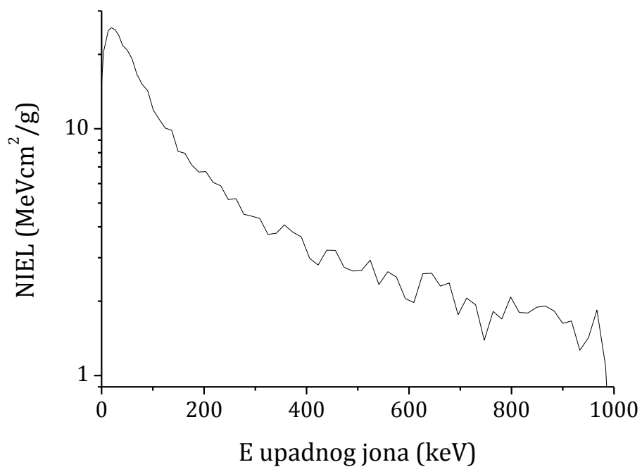
Slika 6.24d. Nejonizujući energetske gubici za alfa čestice u ASS materijalu u zavisnosti od energije.
