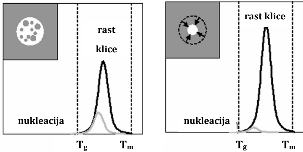
Slika 3.33. Verovatnoća za nukleaciju i rast kao funkcija temperature i prikaz amorfnih tragova u kristalnom fazno promenljivom sloju. a) kristalizacija se odvija kroz dva procesa: nukleacije i rasta klice, b) kristalizacija se događa kroz rast kristala od amorfno-kristalne granične površine ka unutrašnjosti amorfne regije [19].
