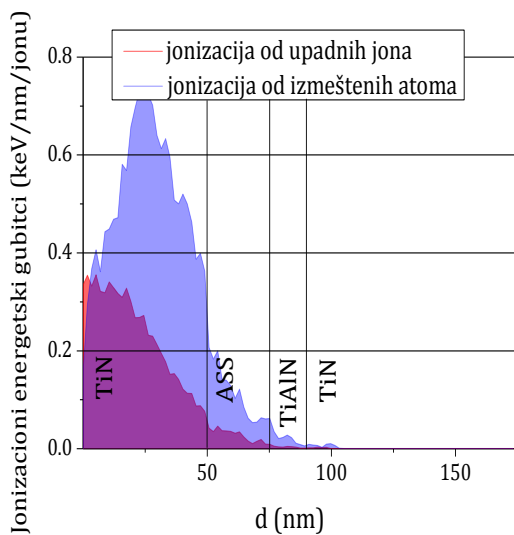
Slika 6.25b. Jonizacioni energetski gubitci nastali od upadnih Fe jona i izmeštenih atoma ćelije FPM-a.
