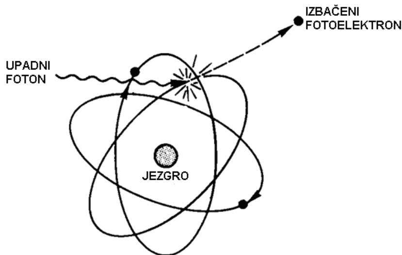
Slika 2.3. Fotoelektrični efekat
