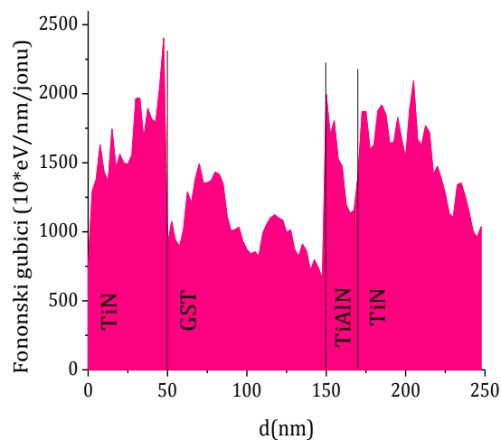
Slika 6.10e. Fononski gubici nastali od upadnih Fe jona i izmeštenih atoma ćelije FPM-a.
