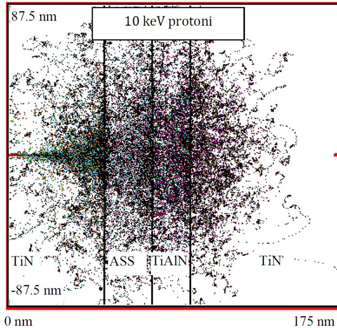
Slika 6.17a. Transport protona kroz fazno promenljivu ćeliju sa ASS slojem.
